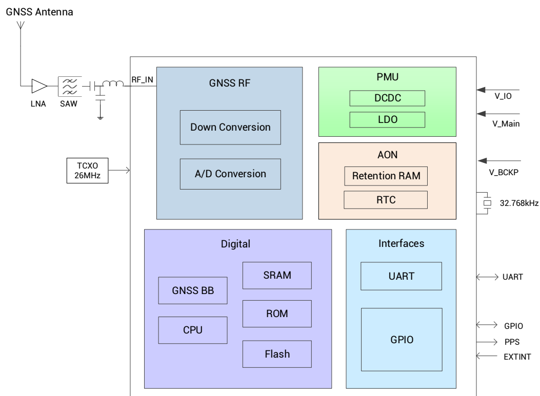
图 1-2 UC6226NIS-E2 芯片框图
