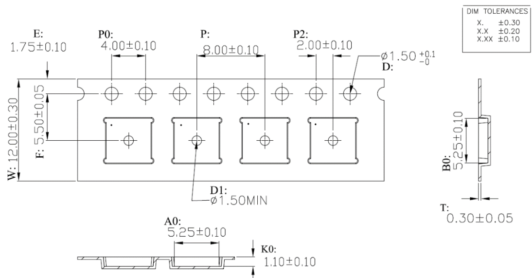
图 11-3 UC6226NIS-E2 编带包装
